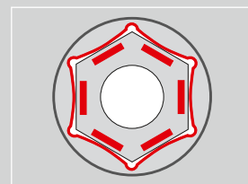
Driver-systém: Krútiaci moment je prenášaný na boky hlavičiek skrutiek a matic, nie do rohov.
